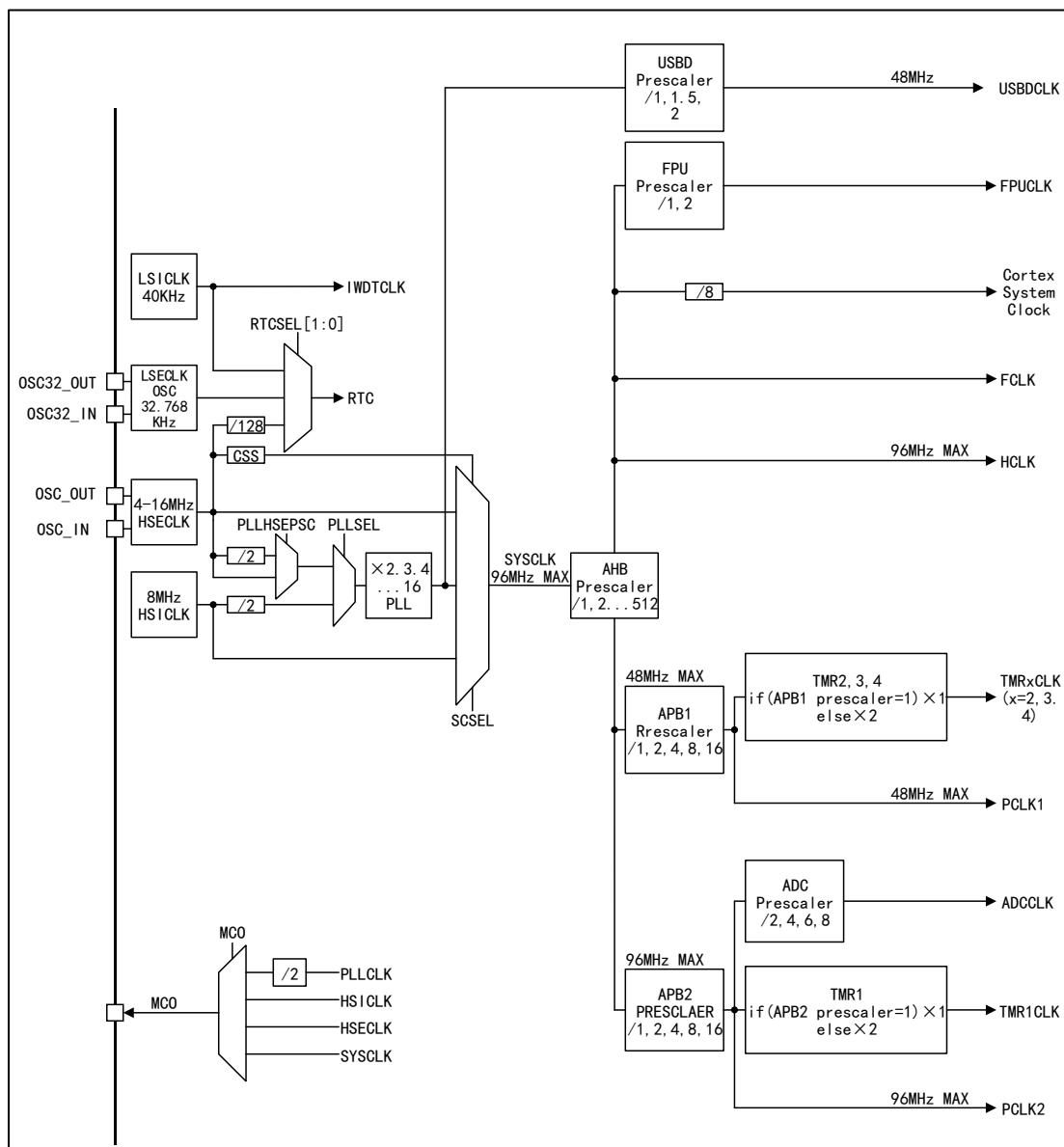
图 3 APM32A103CBT7 时钟树
