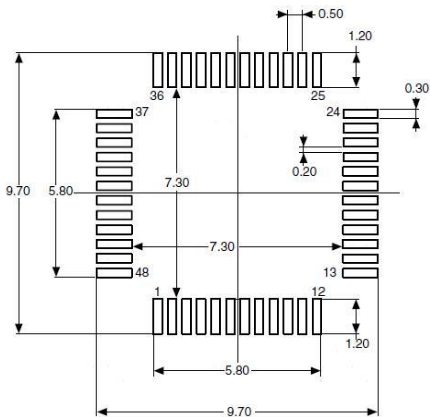
图 14 LQFP48 焊接 Layout 建议
