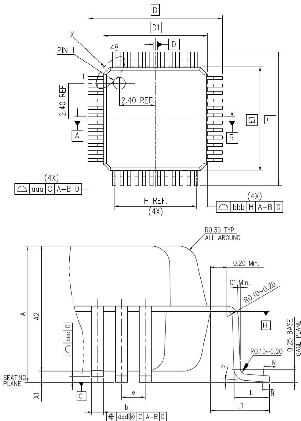
图 13 LQFP48 封装图
